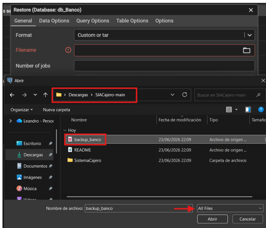
Ilustración 8 Selección de archivo de restauración
